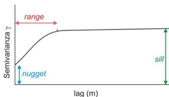
Figura 42. Il variogramma e i suoi parametri principali : nugget cioè l'intersezione della curva con l'asse delle ordinate, costituisce la variabilità casuale non correlata alla distanza; il sill è il valore limite raggiunto dal variogramma una volta esaurita la correlazione fra semivarianza e distanza; il range è la distanza oltre la quale la variabile non mostra più una significativa correlazione spaziale.
